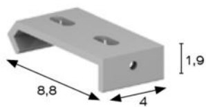
PIASTRA IN ALLUMINIO A SCOMPARSA
