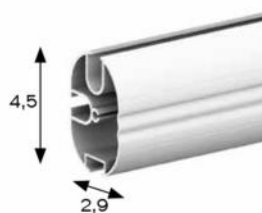
TERMINALE ④
