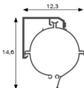
ATTACCO PARETE
