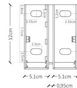
VISTA FRONTALE
