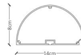
PROFILO TRAVE TETTINO
