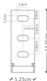
VISTA FRONTALE
