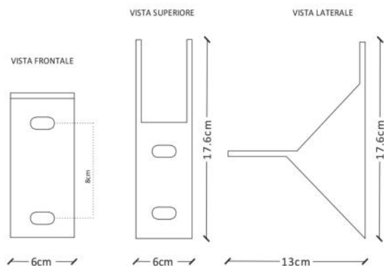
STAFFA ANCORAGGIO A SOFFITTO SINGOLA
