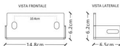
STAFFA ATTACCO TRAVE LATERALE A MURO
