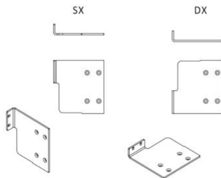
ATTACCO TRAVE LATERALE SU GRONDA
