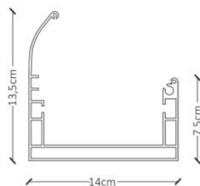
GRONDA
