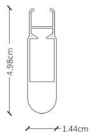
PROFILO CAPPOTTINA
