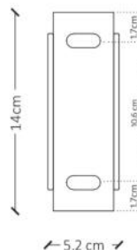
PIEDE REGOLABILE
