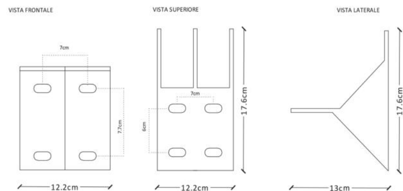
STAFFA ANCORAGGIO A SOFFITTO DOPPIA
