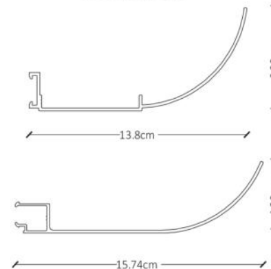
CASSONETTO A/B
