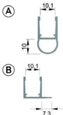
A) GUARNIZIONE CENTRALE E/O LATERALE B) GUARNIZIONE VETRO/VETRO
