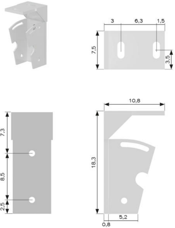
STAFFA A SOFFITTO IN ACCIAIO INOX
