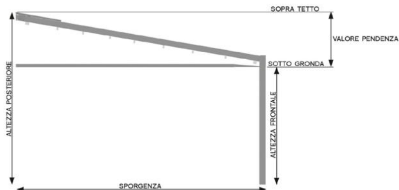
VISTA LATERALE
