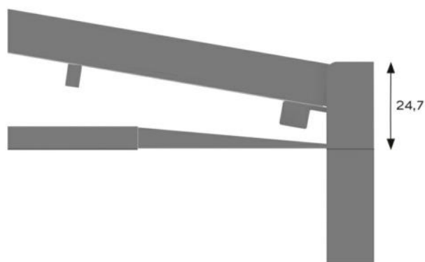
INGOMBRO GRONDA
