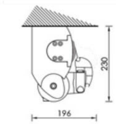
INSTALLAZIONE A SOFFITTO
